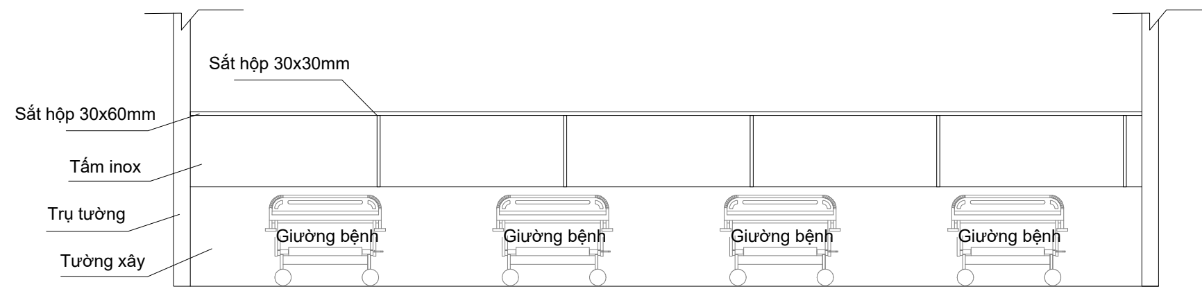
MẶT ĐỨNG CHI TIẾT GIÁ ĐỠ LẮP ĐẶT BHU CT1 LOẠI 4 G DÀI ...M
